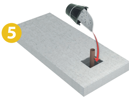
5 Découpe du fond coffrant à l'aide d'une scie cloche / scie sabre au diamètre du futur traversant. Passage de tuyau / gaine à travers le perçement réalisé
